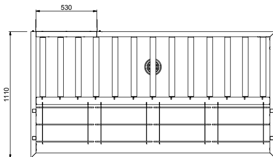
Boven aanzicht
